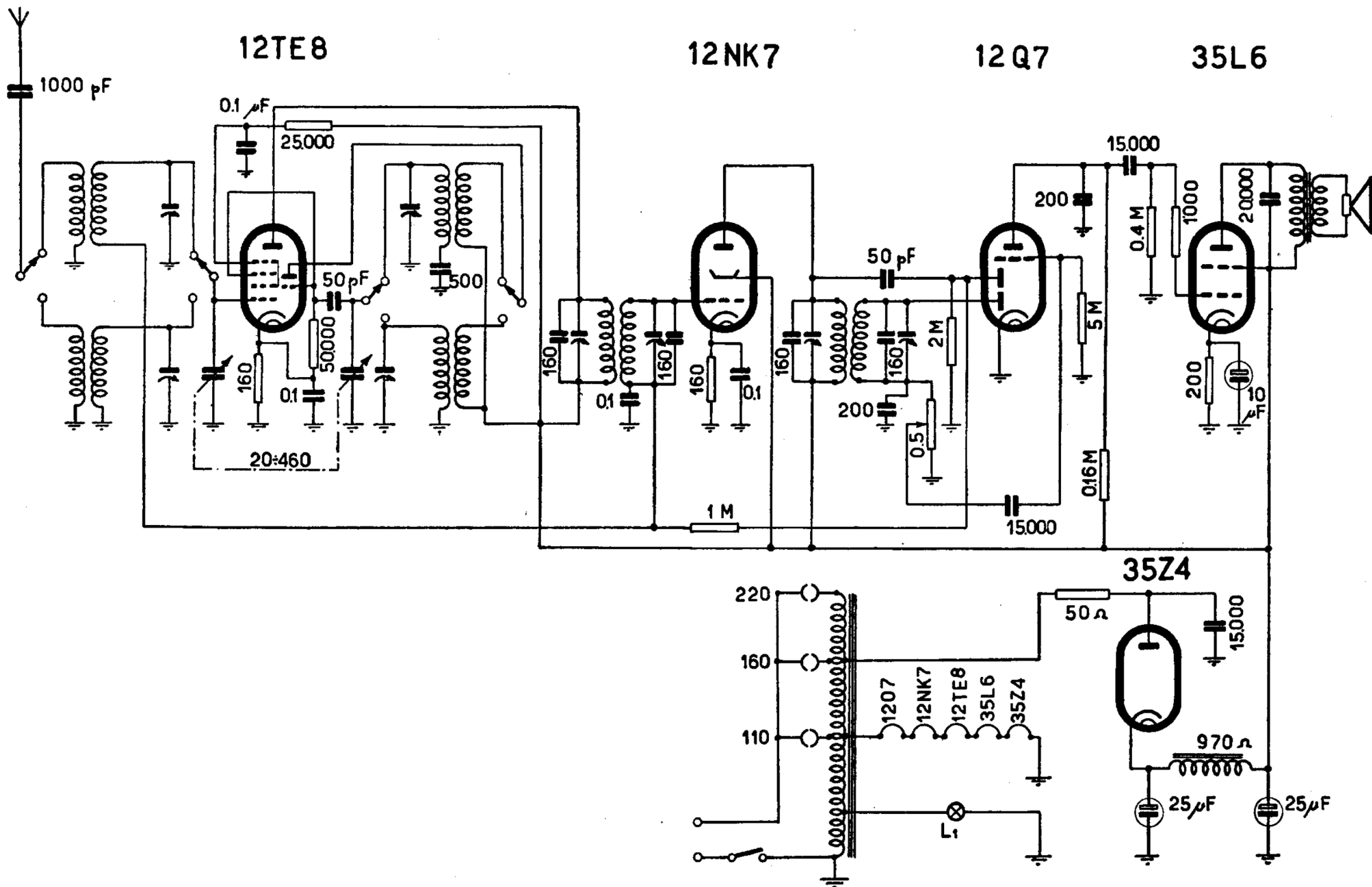
SAFAR - Mod. 527 A - Media frequenza: 450 kc/s. Tensioni: 12TE8 pl. 110, sch. 55, pl. osc. 90, catodo 2. 12NK7 pl. 110, sch. 110, gr. 2, 12Q7 pl. 70, 35L6 pl. 100, sch. 110, gr. 6. 35Z4 pl. 160 V c. a. Taratura v. tabella a parte.
